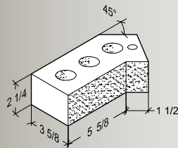
45° Dogleg
