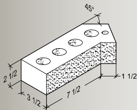
45° Dogleg
