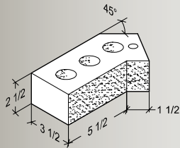
45° Dogleg
