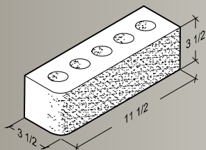
3\frac{1}{2} \times 3\frac{1}{2} \times 11\frac{1}{2} Bullnose
