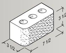
3\frac{1}{2} \times 3\frac{1}{2} \times 7\frac{1}{2} 2 Bullnose Face
