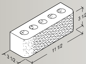
3\frac{1}{2} \times 3\frac{1}{2} \times 11\frac{1}{2} 2 Bullnose Face
