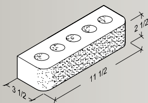
3\frac{1}{2} \times 2\frac{1}{2} \times 11\frac{1}{2} 2 Bullnose Face
