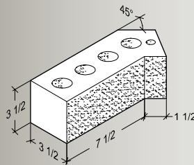
45° Dogleg
