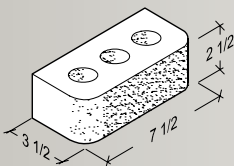
3\frac{1}{2} \times 2\frac{1}{2} \times 7\frac{1}{2} 2 Bullnose Face
