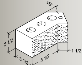
45° Dogleg
